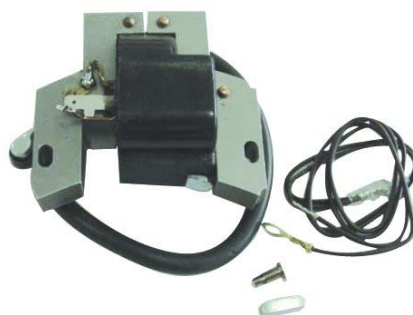
Elektronisk tændspole Passer til Briggs og Stratton 2-4 hk. Lodret/vandret. Erstatter OEM nr. Briggs og Stratton: 398593, 496914, John Deere: PT11047.
