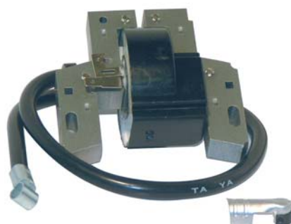
Elektronisk tændspole Passer til Briggs og Stratton Vanguard 9, 12,5 og 14 hk, V-tvin 12, 12,5 hk. Erstatter OEM nr. Briggs og Stratton 490586, 492341, 495859.
