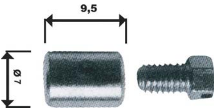
Kabelstop til 2,2 mm Ø7 x 9,5 mm.
